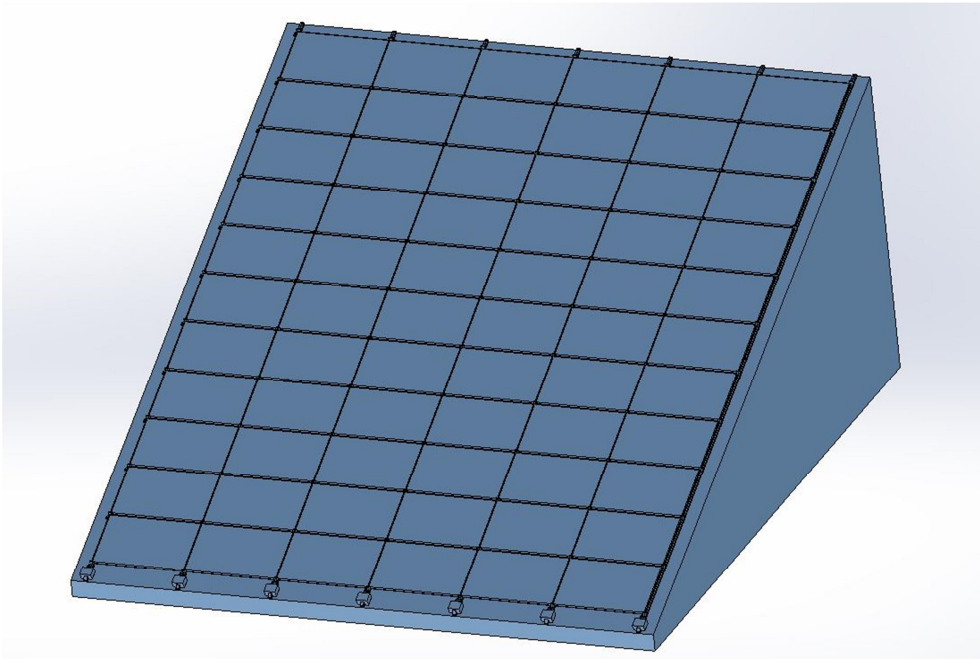
Bild 1.1: Isometrische Ansicht einer Feldanordnung des dachparallelen PV-Systems ILZOCLIP auf einem Pultdach mit 25° Dachneigung
